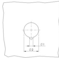
Verkleidungsbohrung
